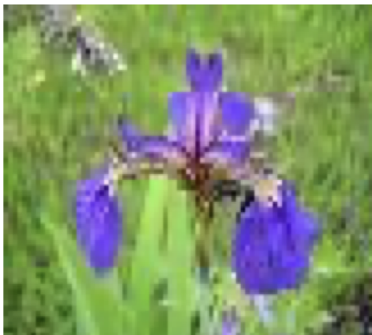
Рисунок 1 – Ирис setosa
